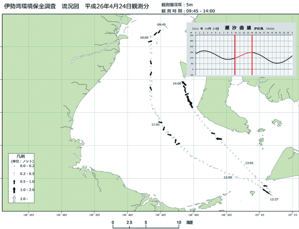
Fig. 2. Result of current observation in April 24, 2014. 図2. 流況調査結果 (平成 26 年 4 月 24 日).
