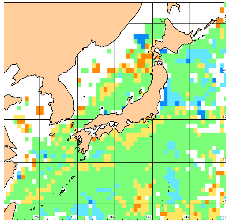
2003年2月水温平年差
