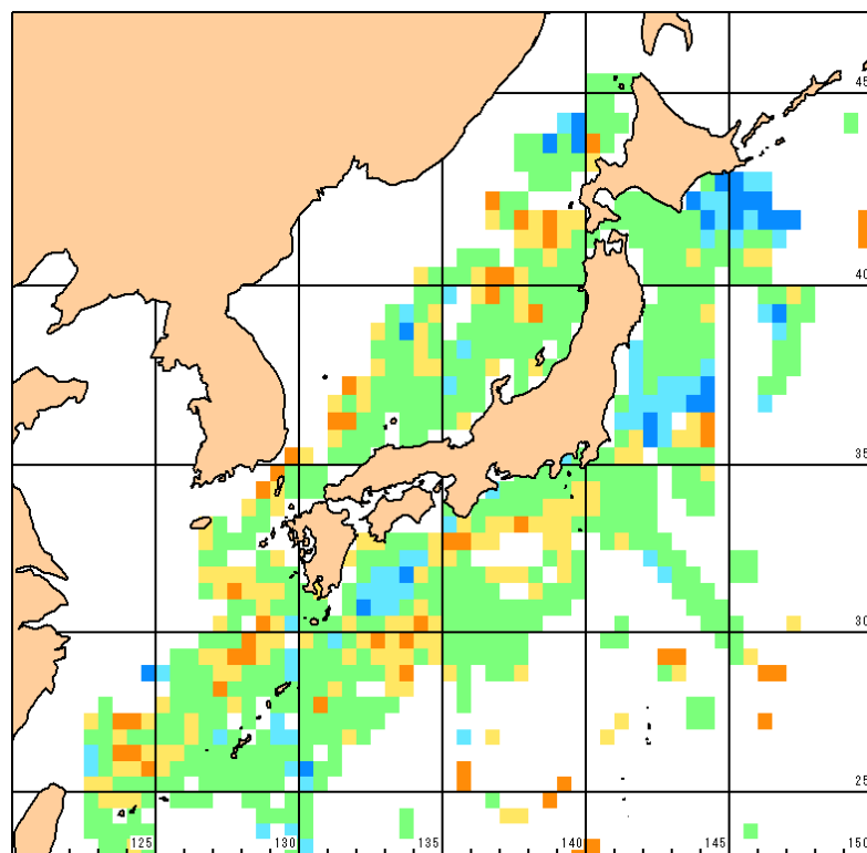
2003年2月水温平年差
