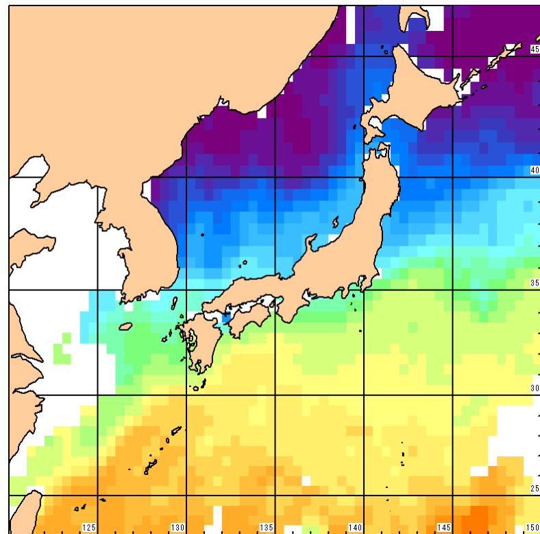
2月の水温平年値( ) 日本海洋データセンターの統計値
