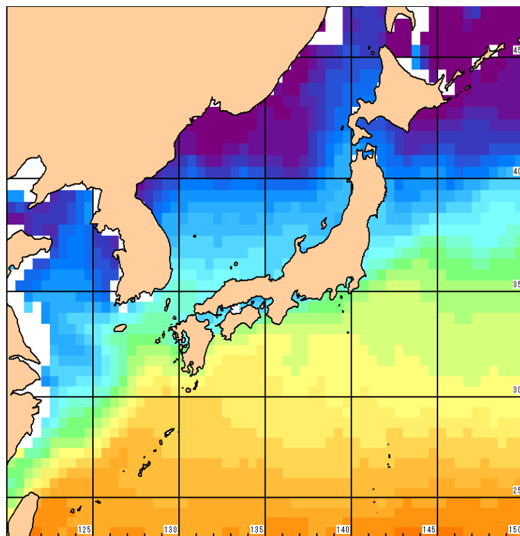
2月の水温平年値( ) 日本海洋データセンターの統計値
