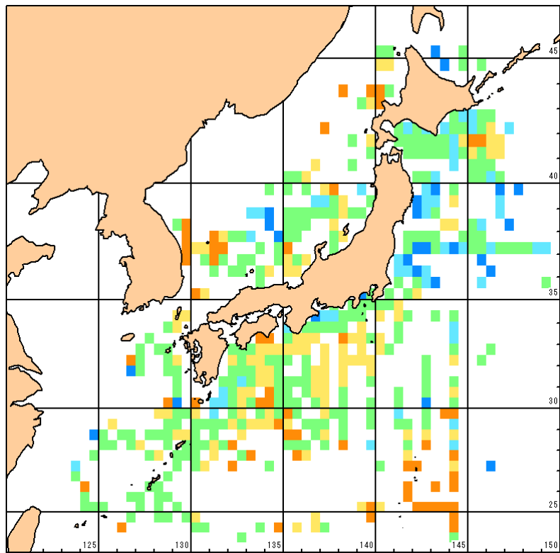
2004年2月水温平年差
