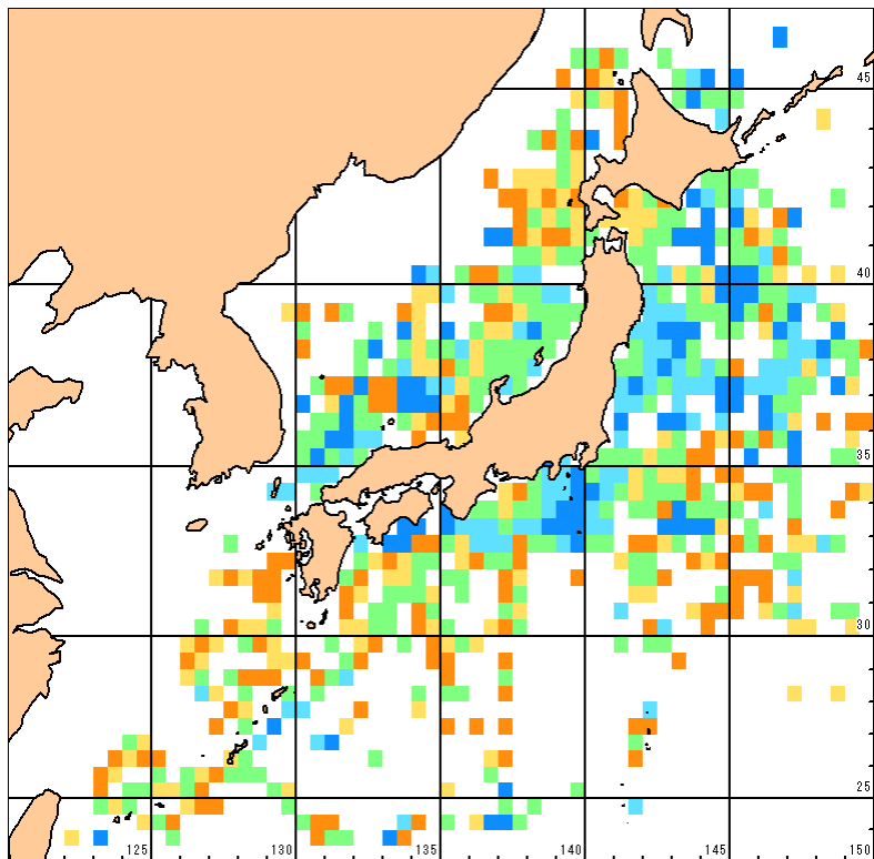
2005年7月水温平年差
