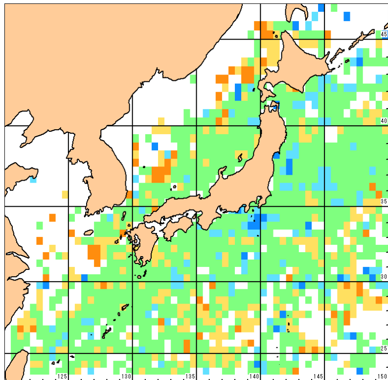
2005年7月水温平年差
