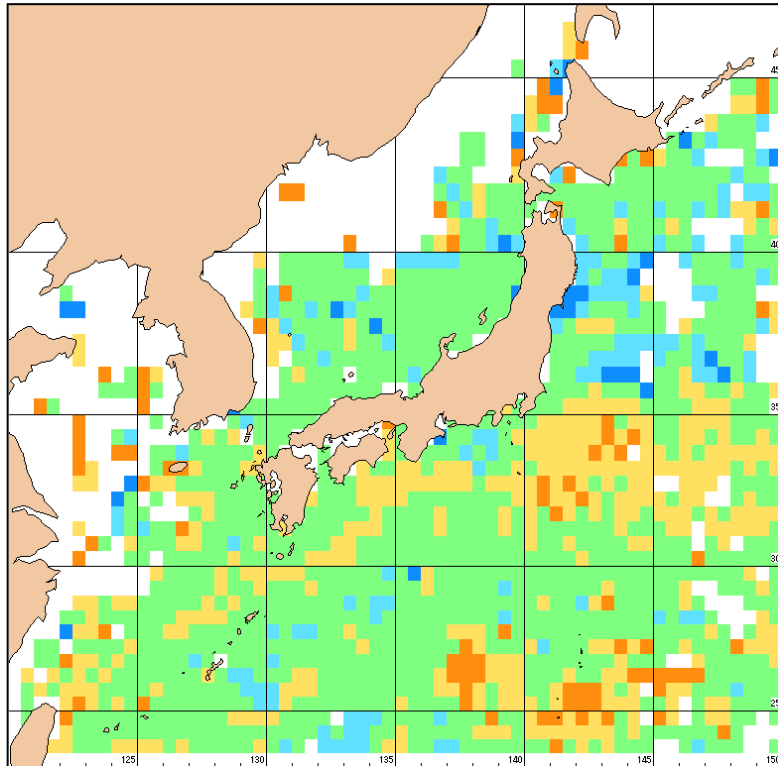
2006年3月水温平年差
