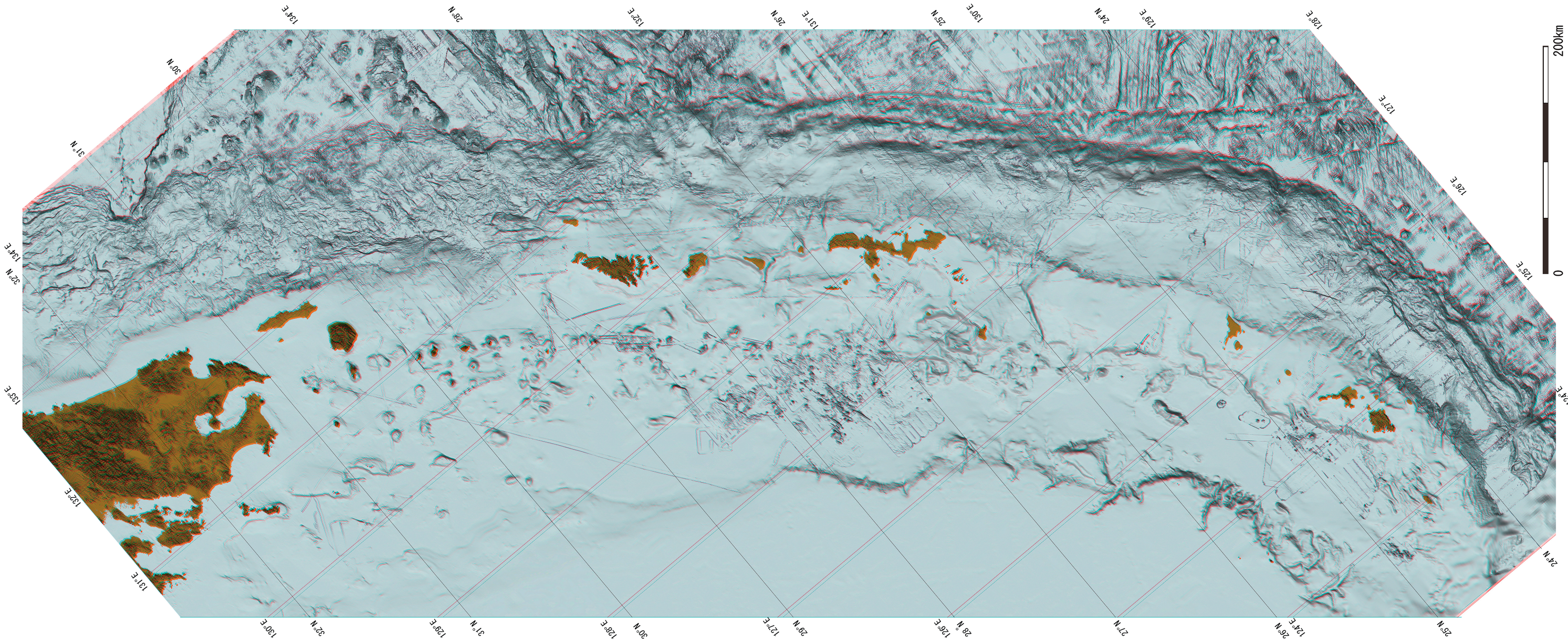
Appendix Anaglyph image along Nansei-Shoto Trench. 付図. 南西諸島海溝沿いのアナグリフ画像.
